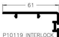
P10119 INTERLOCK
